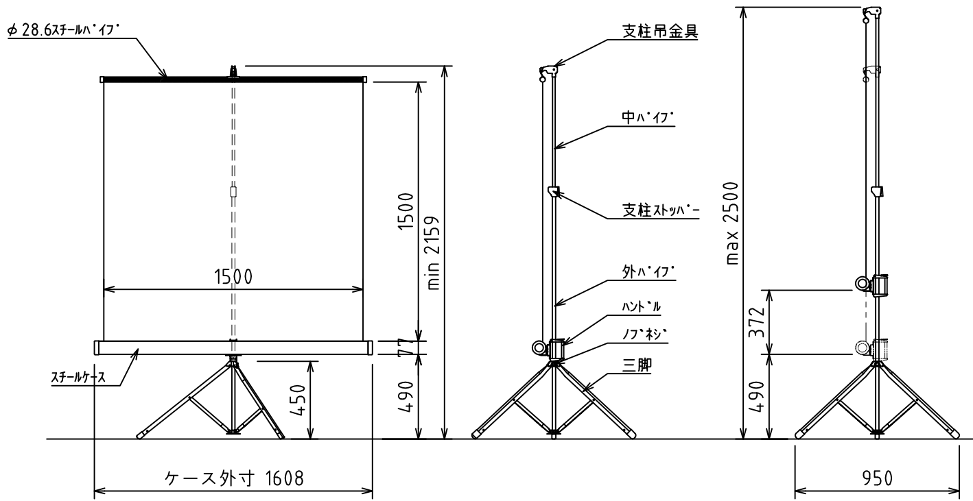
外観図 1/30
