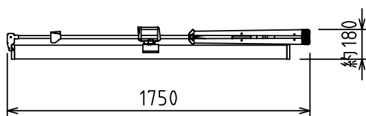
脚収納図
