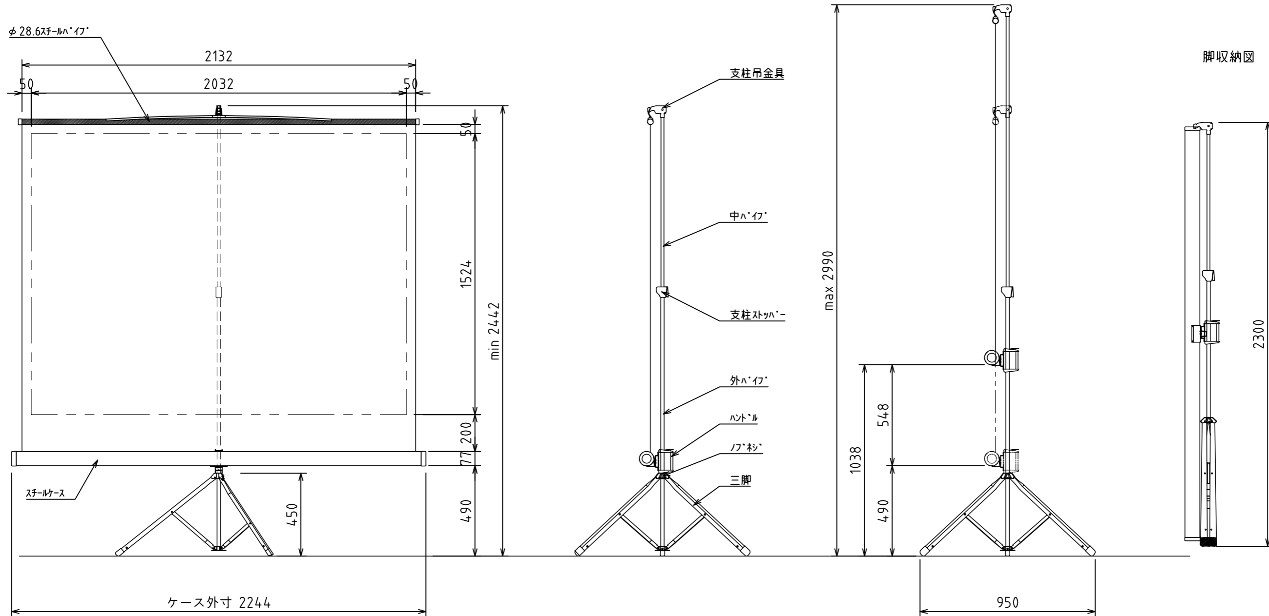
外観図 1/20
