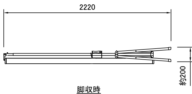
外観図 S=1/30
