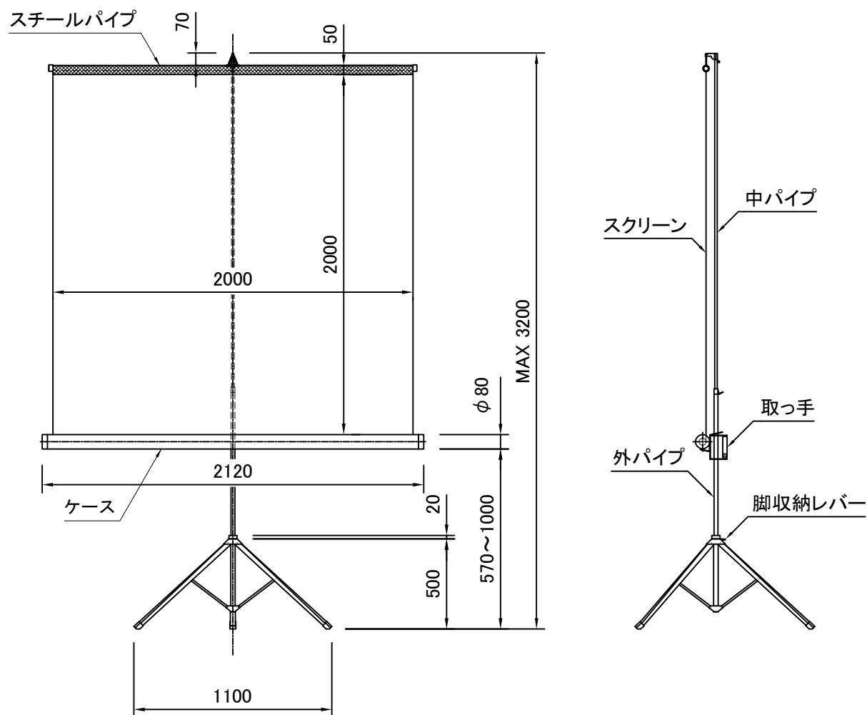
外観図 S=1/30
