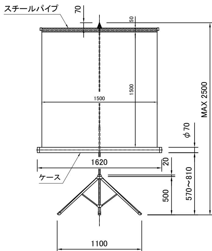
外観図 S=1/30
