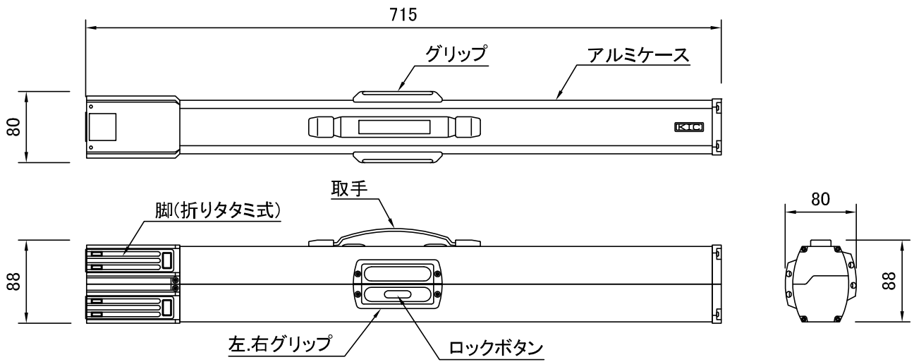
スクリーン収納時ケース外寸 S=1/6
