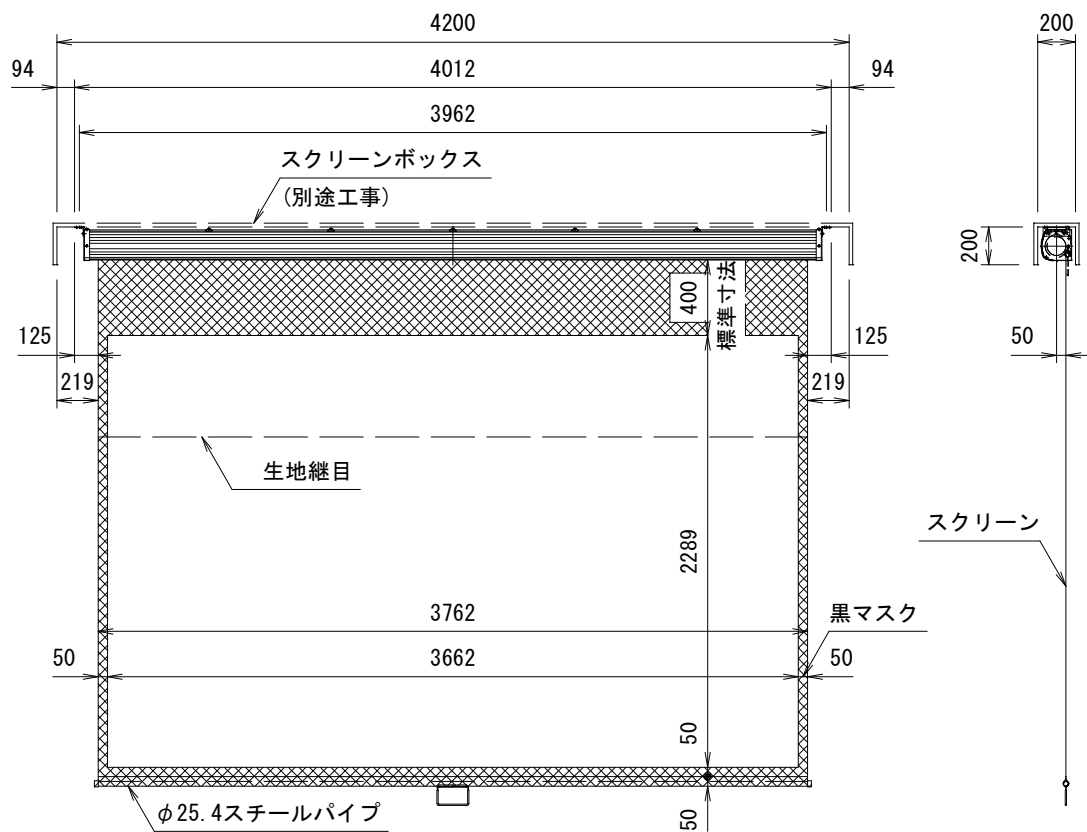
外観図 S=1/40
