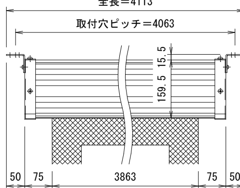
取付部詳細図 S=1/10
