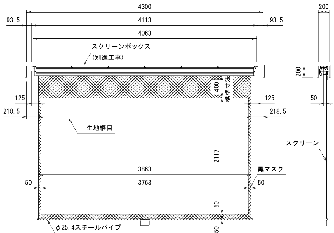
外観図 S=1/40
