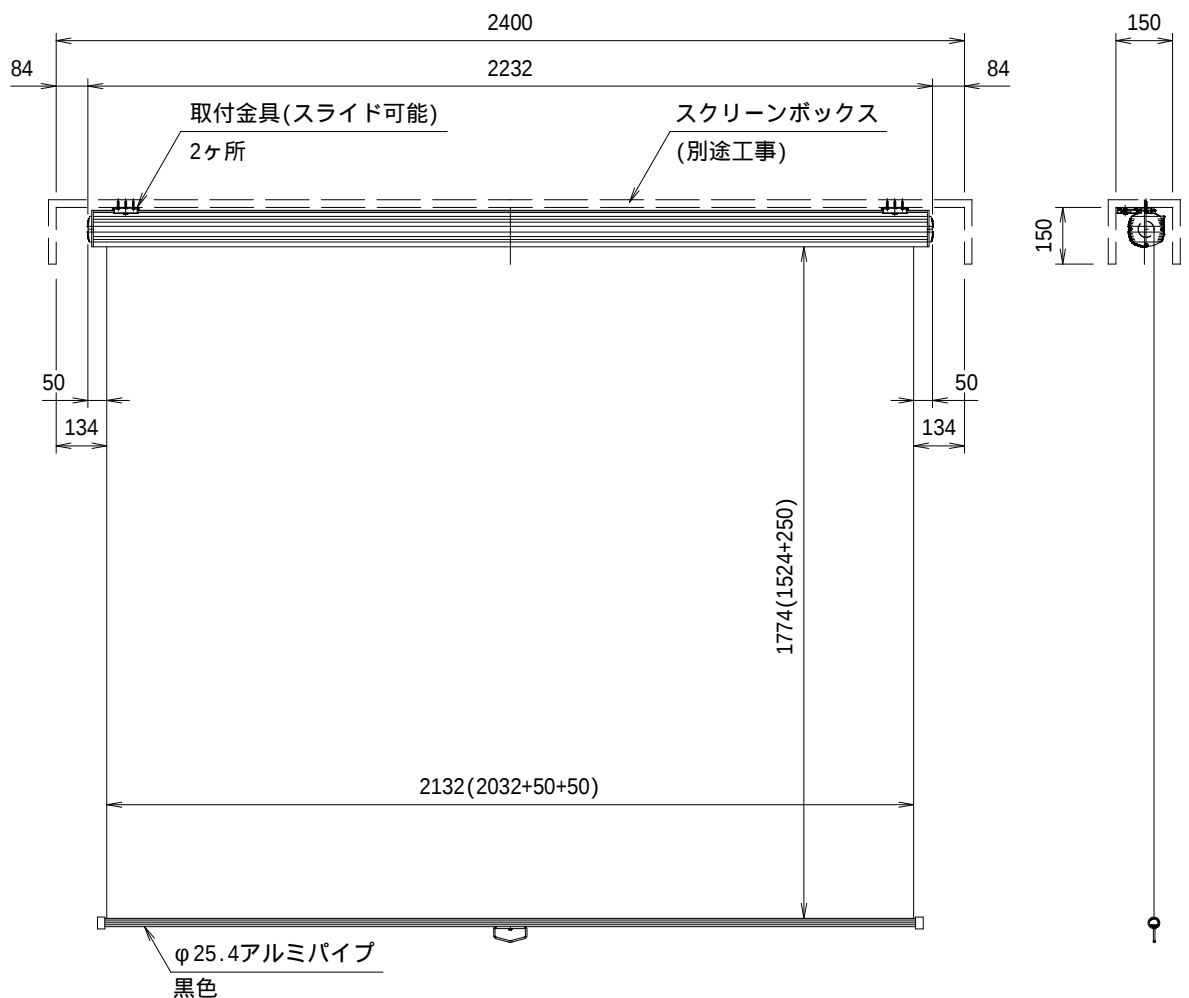
外観図 S=1/20
