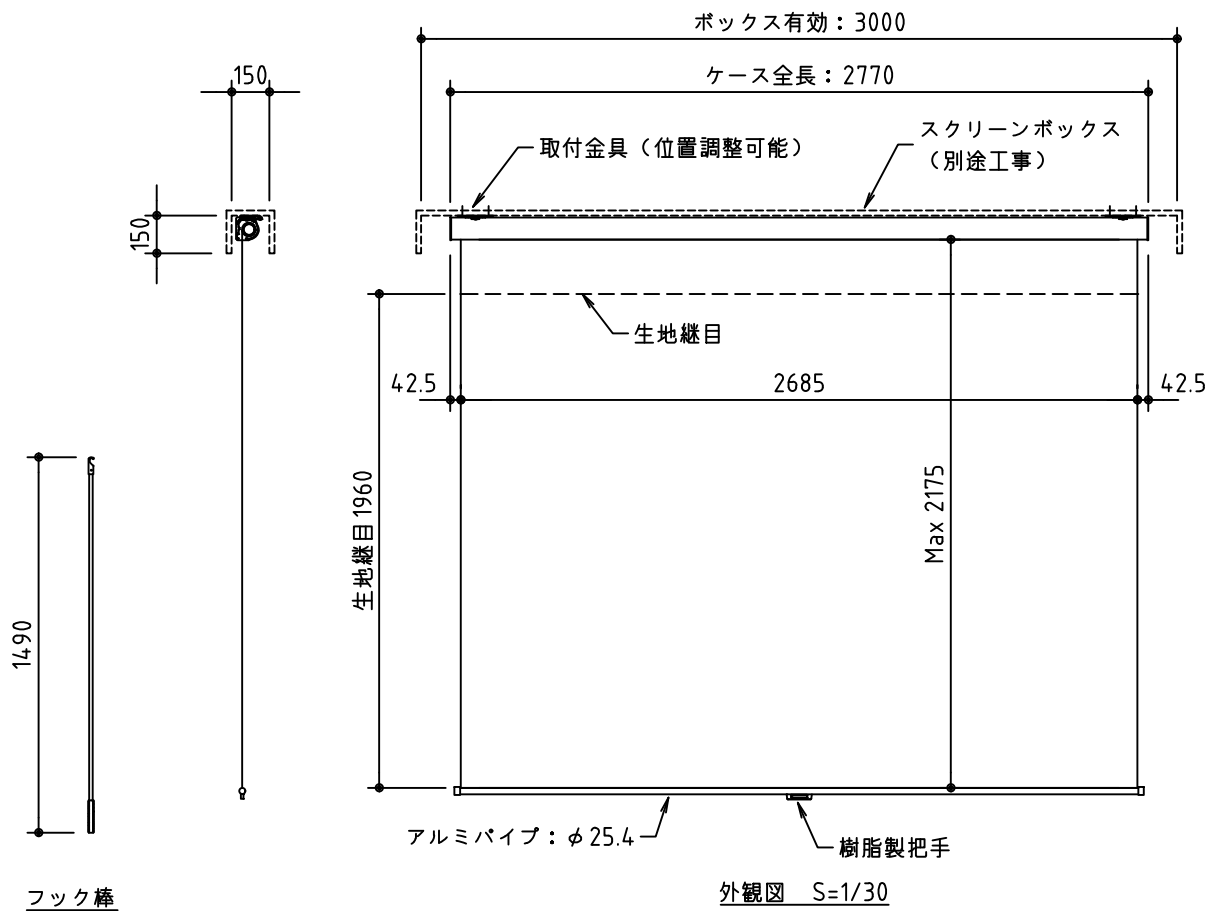
外観図 S=1/30
