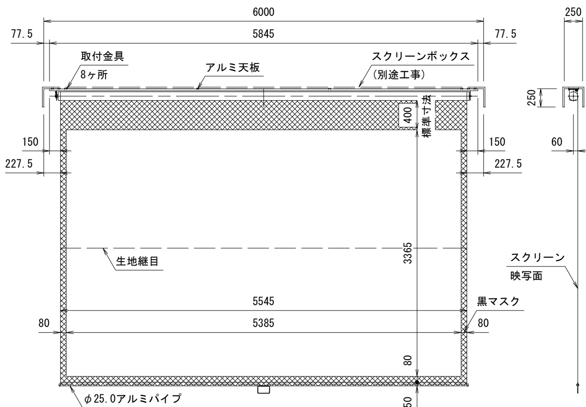
外観図 S=1/50
