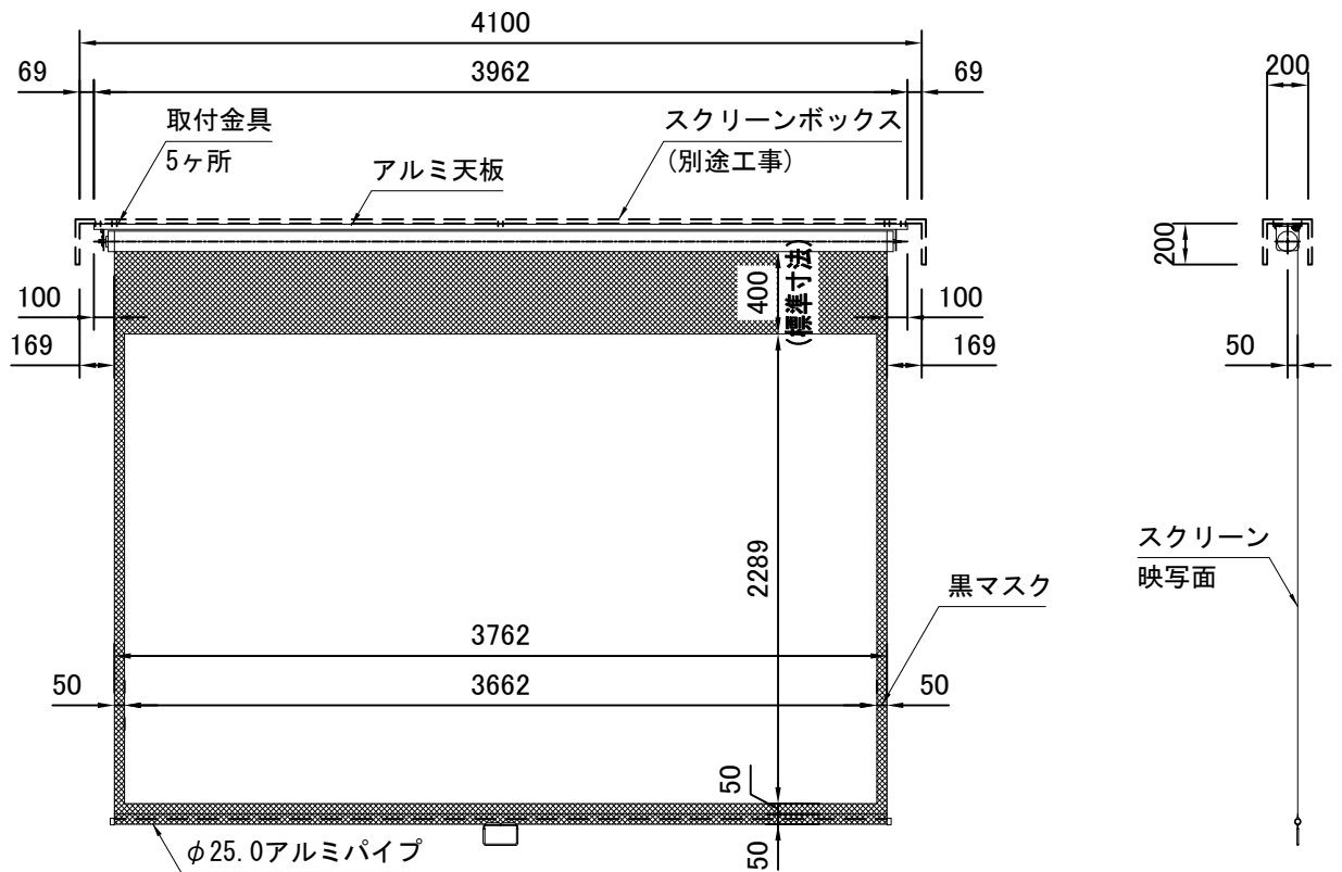
外観図 S=1/40
