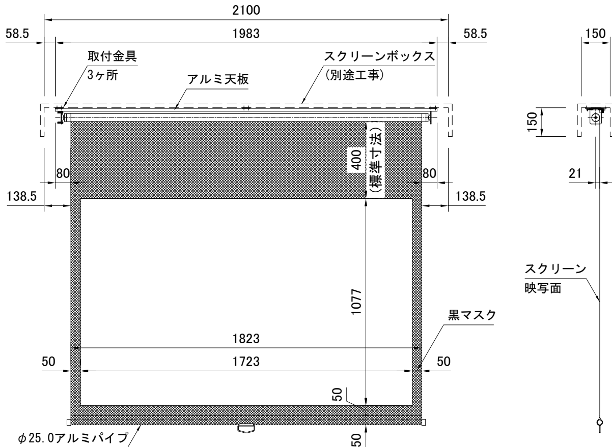
外観図 S=1/20
