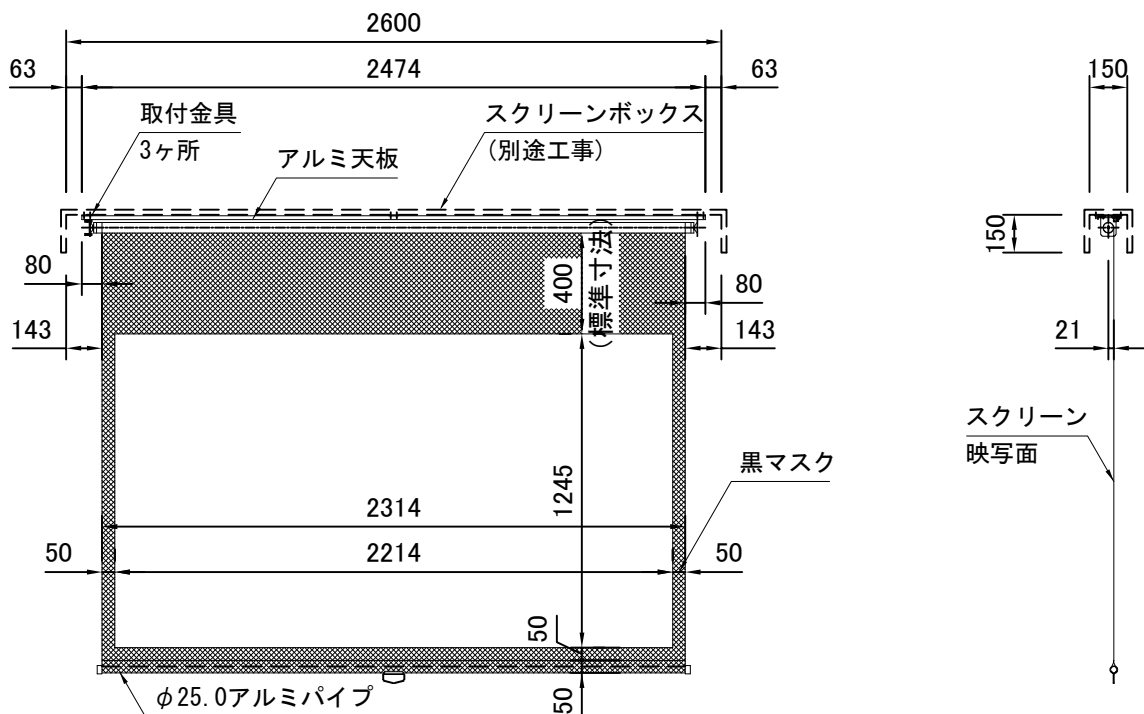
外観図 S=1/30
