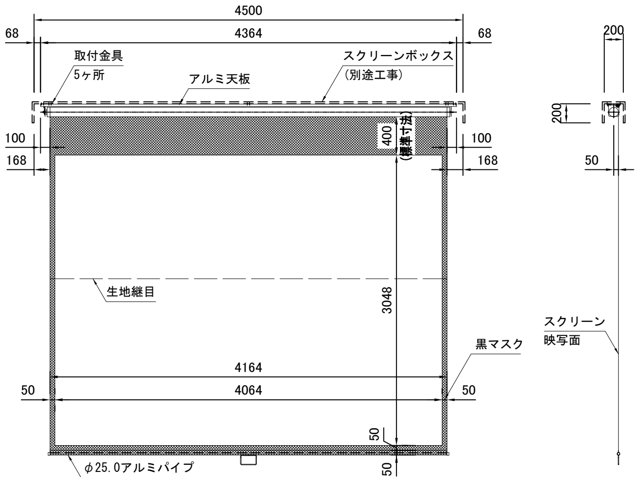
外観図 S=1/40
