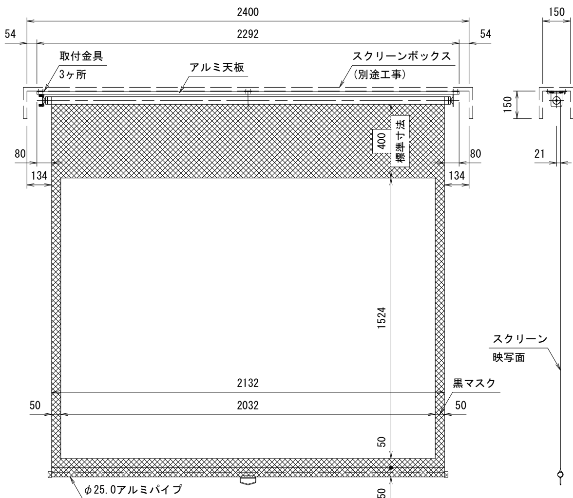
外観図 S=1/20
