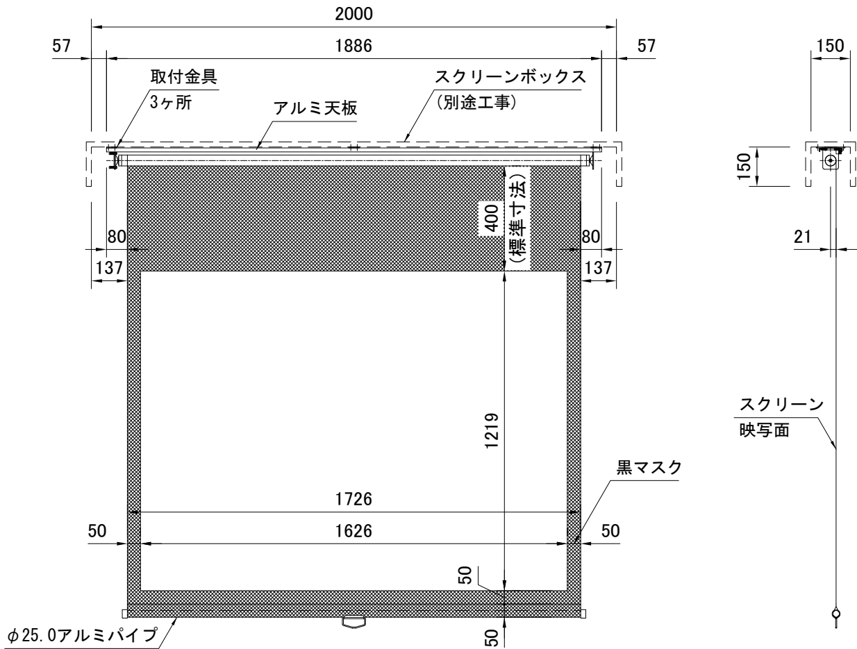
外観図 S=1/20
