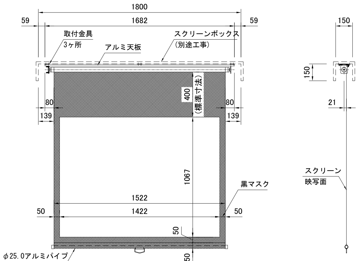
外観図 S=1/20
