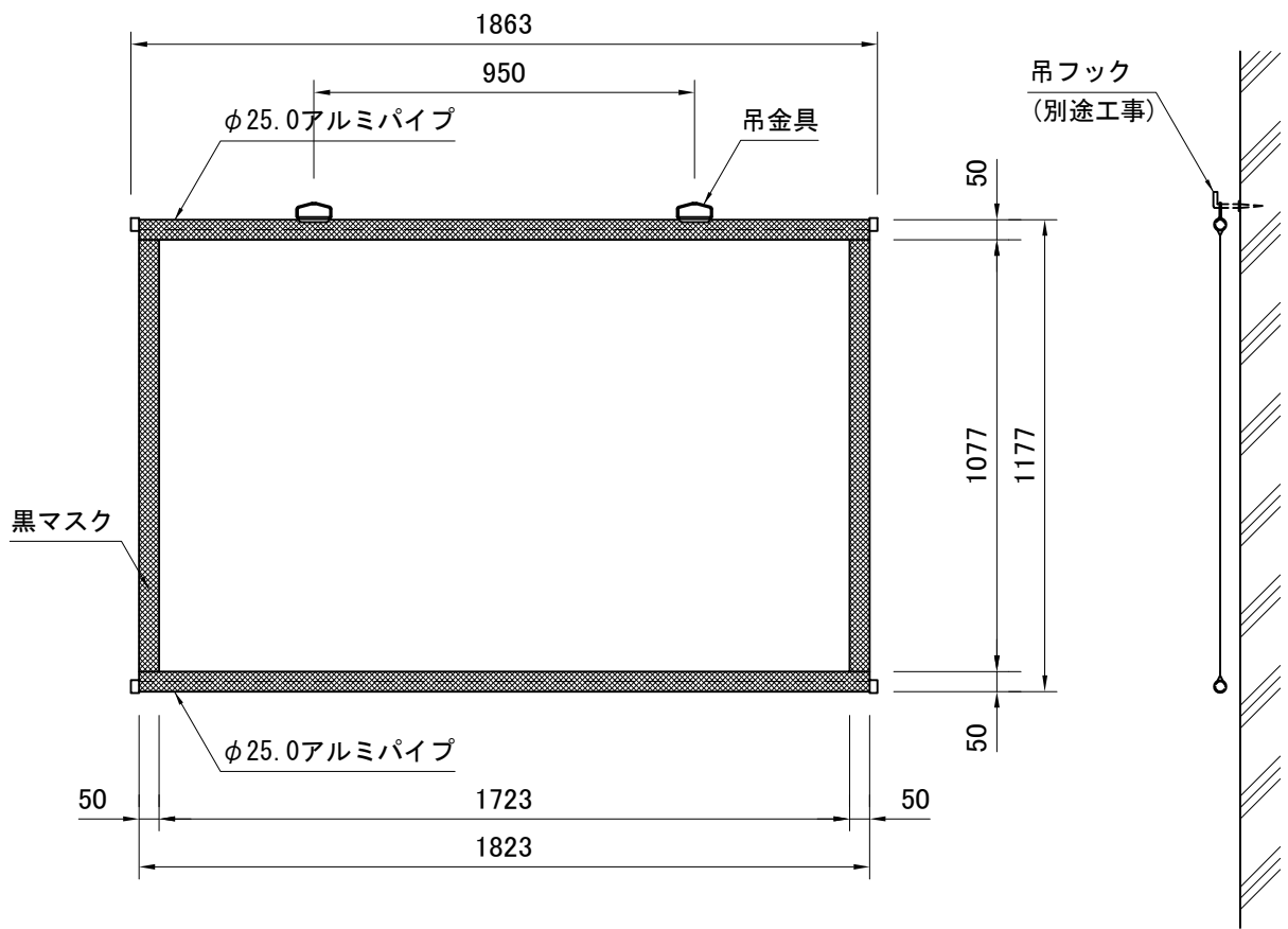
外観図 S=1/20
