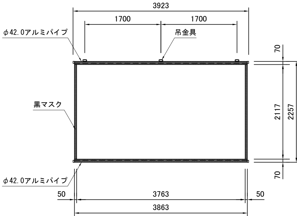
外観図 S=1/50
