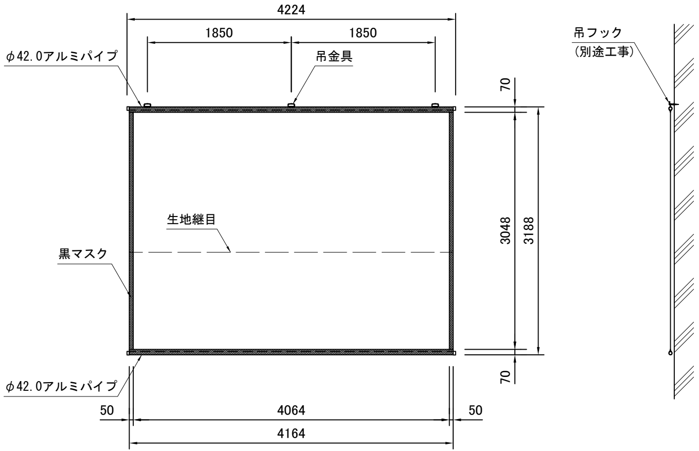
外観図 S=1/50
