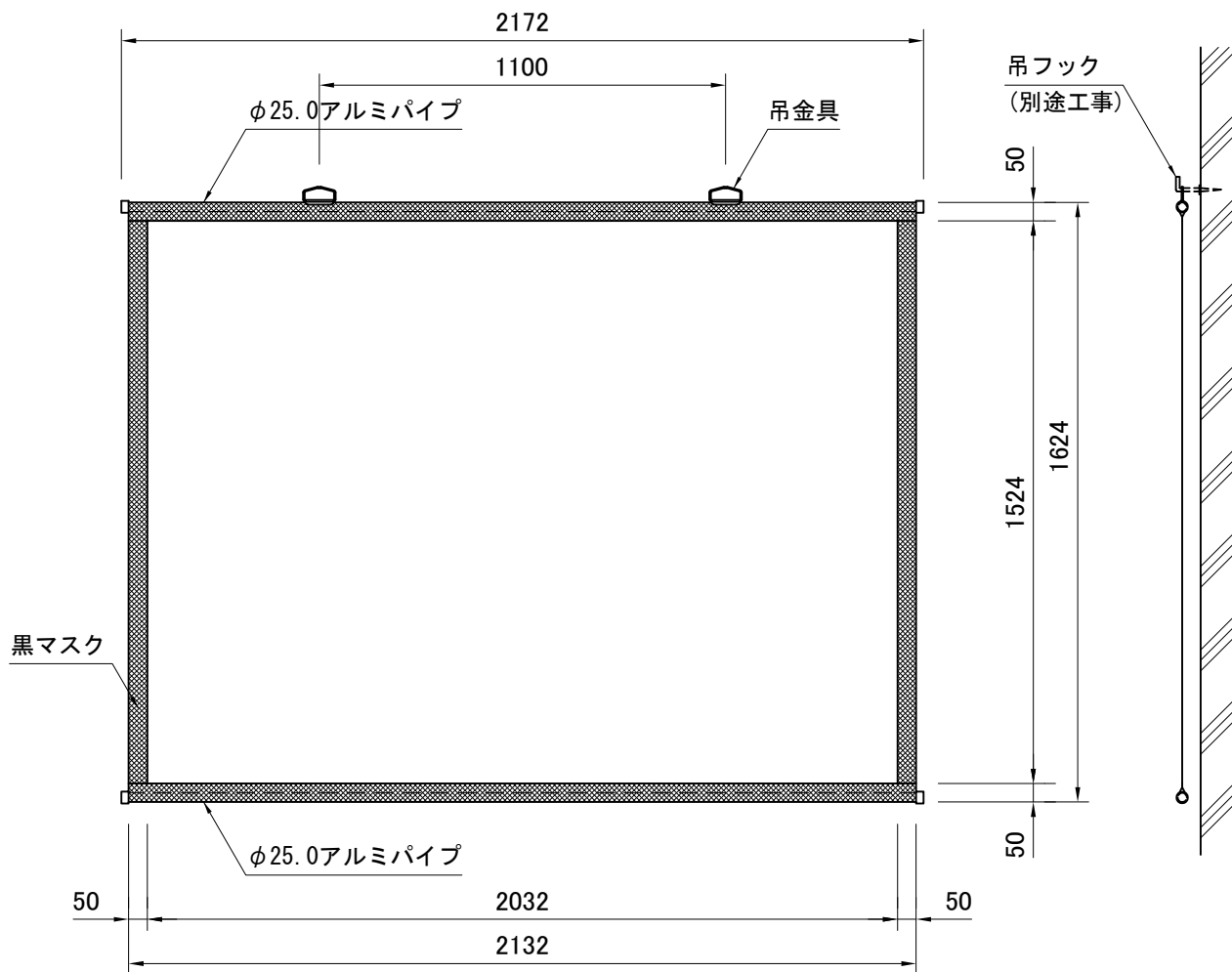
外観図 S=1/20
