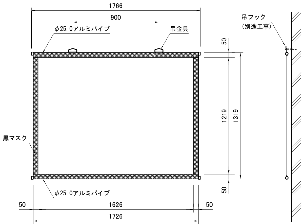
外観図 S=1/20
