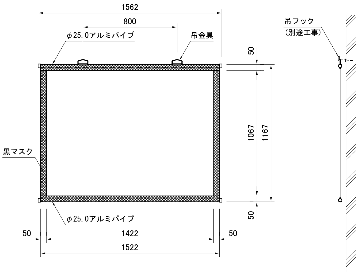
外観図 S=1/20
