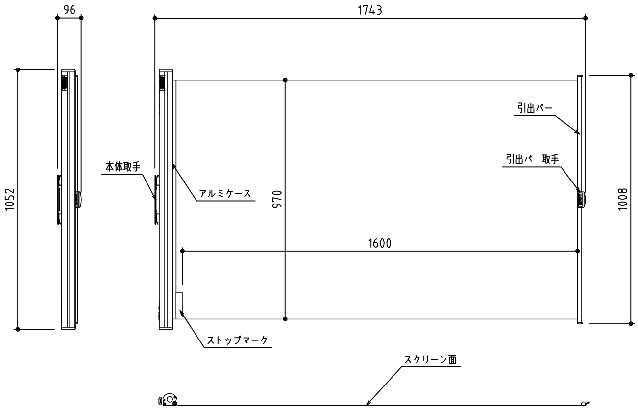
外觀図 S=1/15
