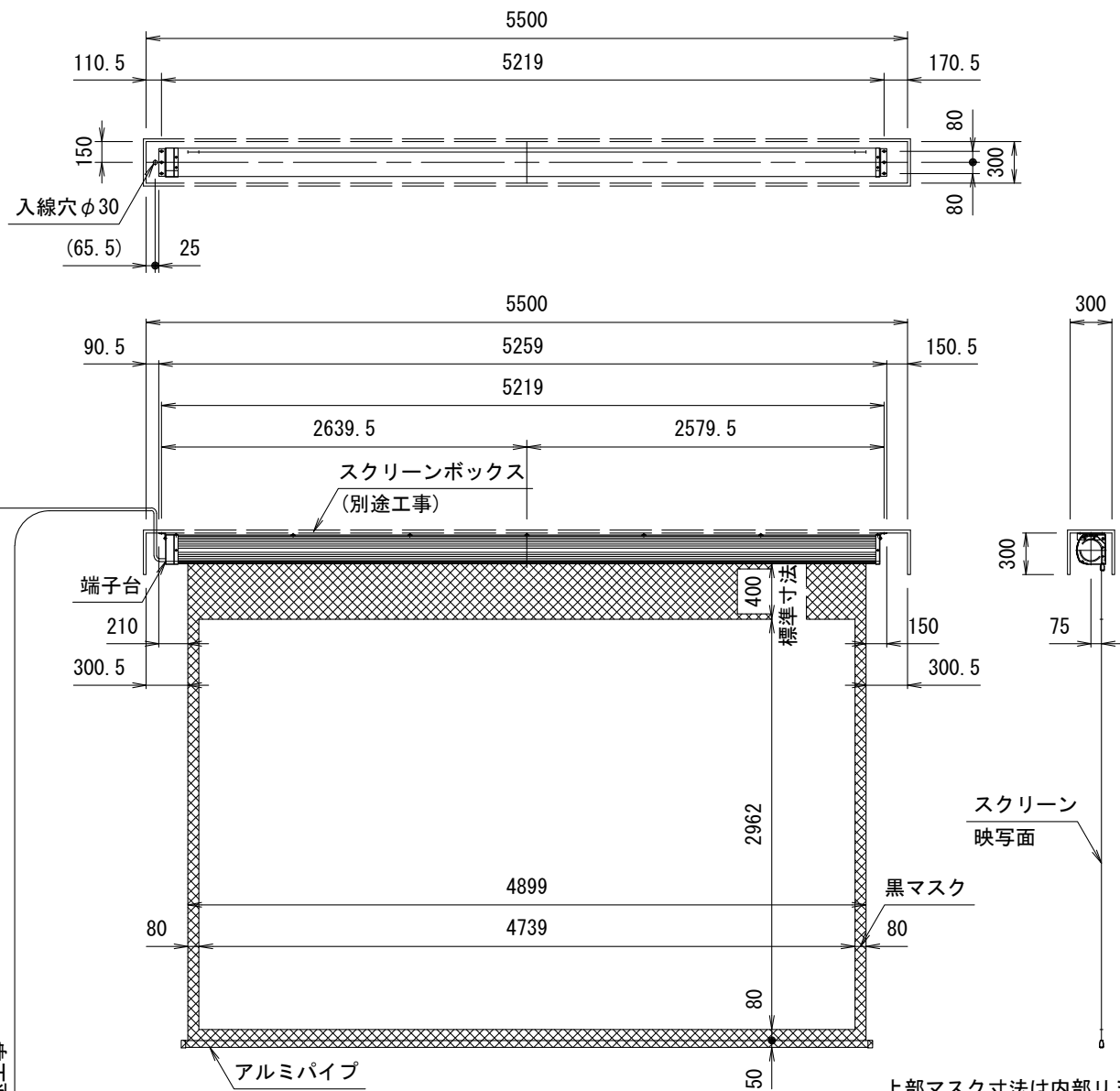
外観図 S=1/50
