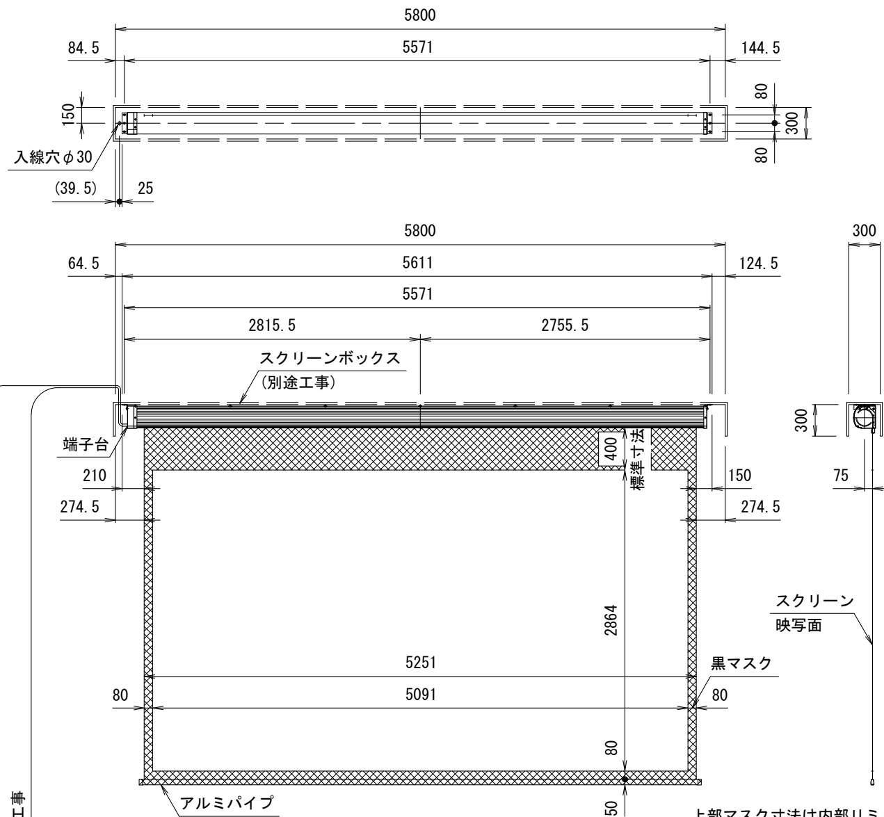
外觀図 S=1/50
