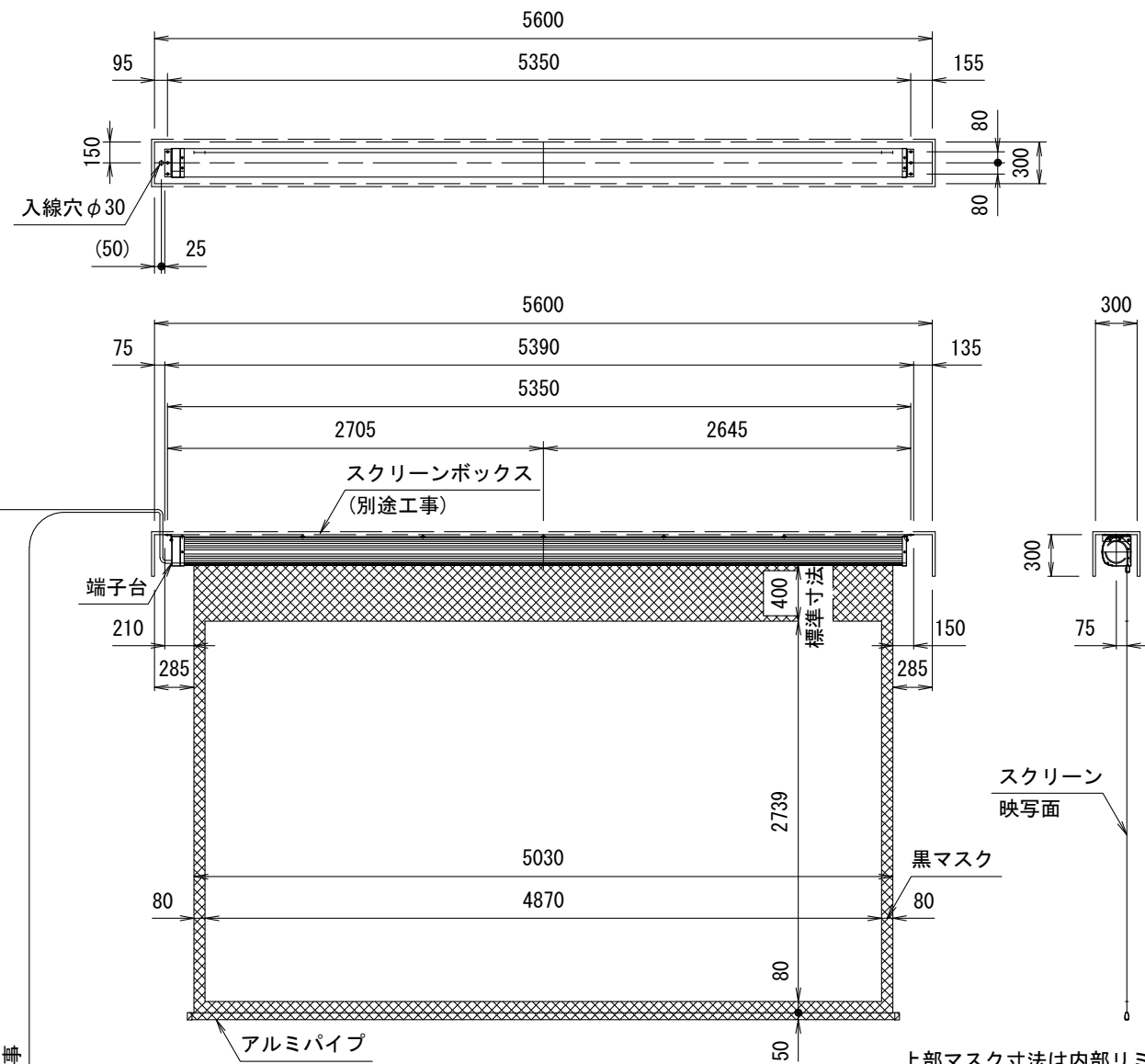
外観図 S=1/50
