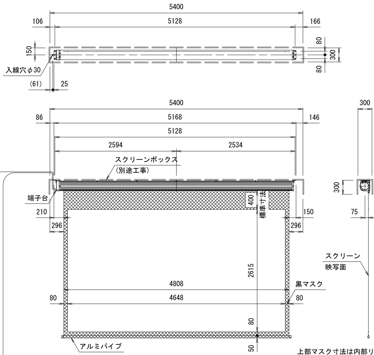
外觀図 S=1/50
