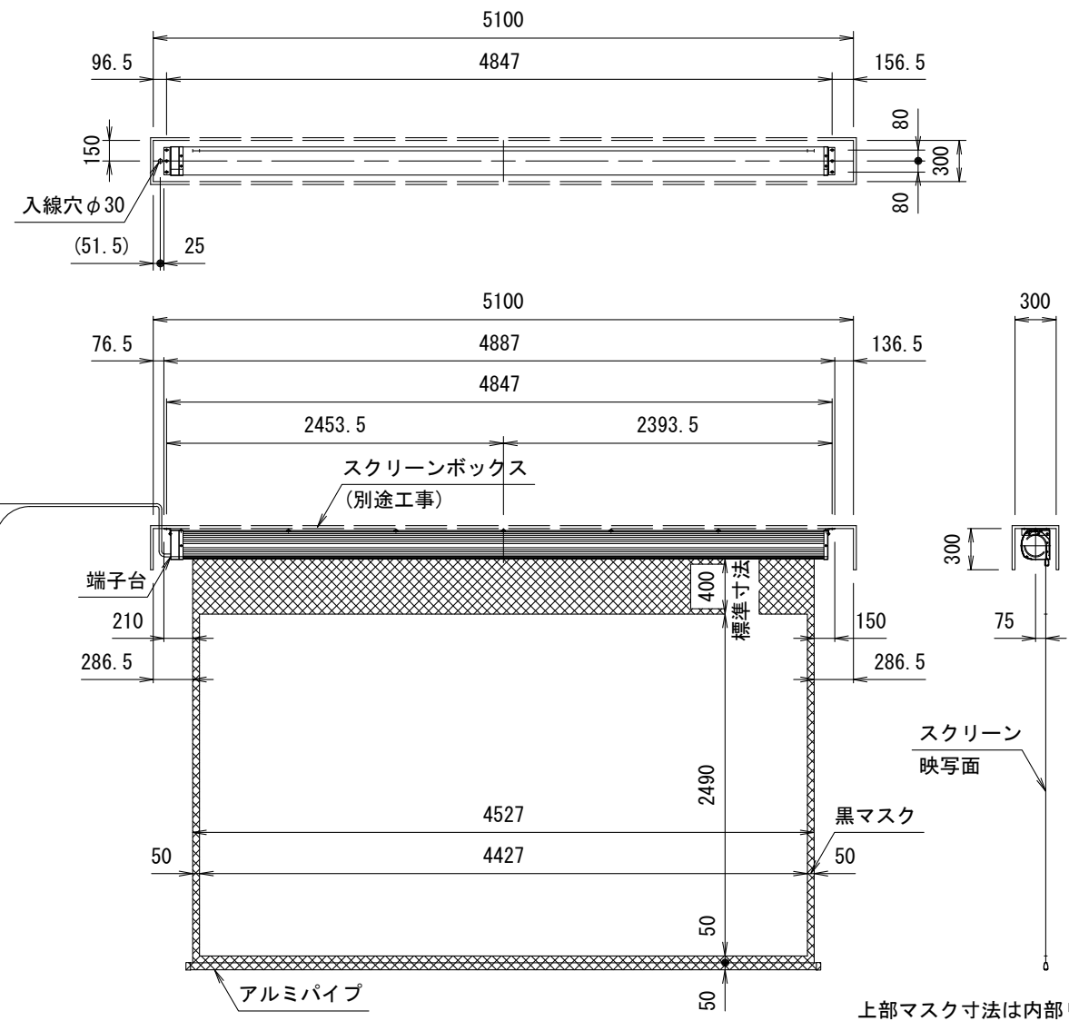
外観図 S=1/50
