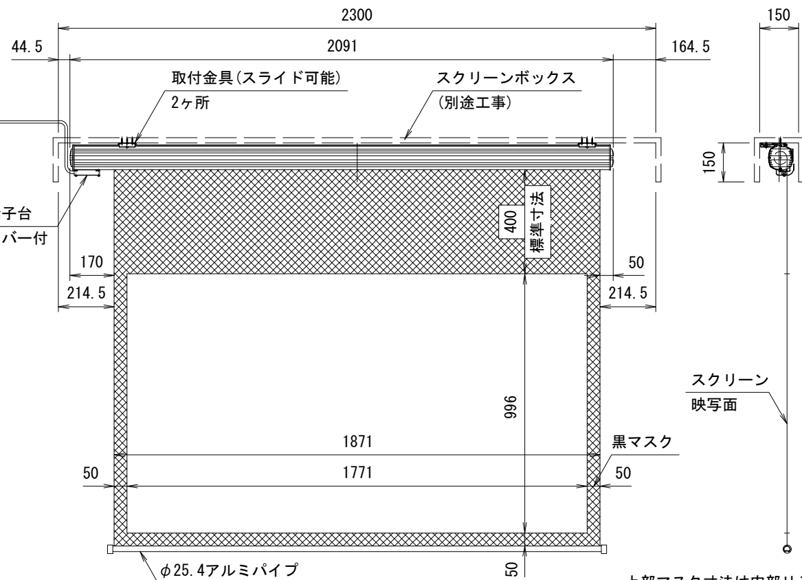
外観図 S=1/20
