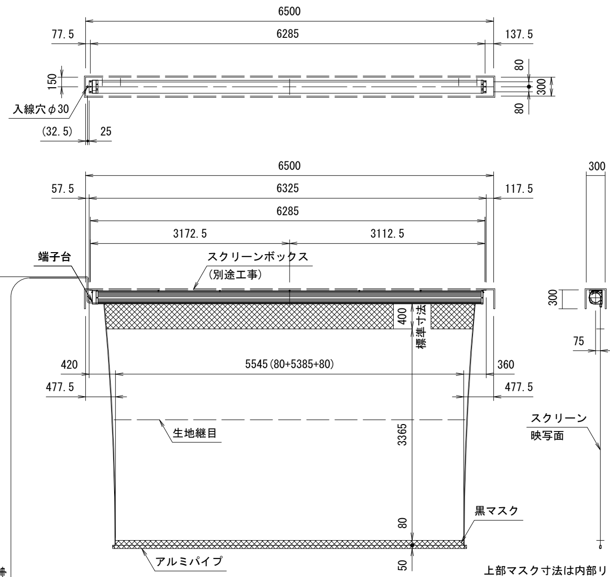
外観図 S=1/60
