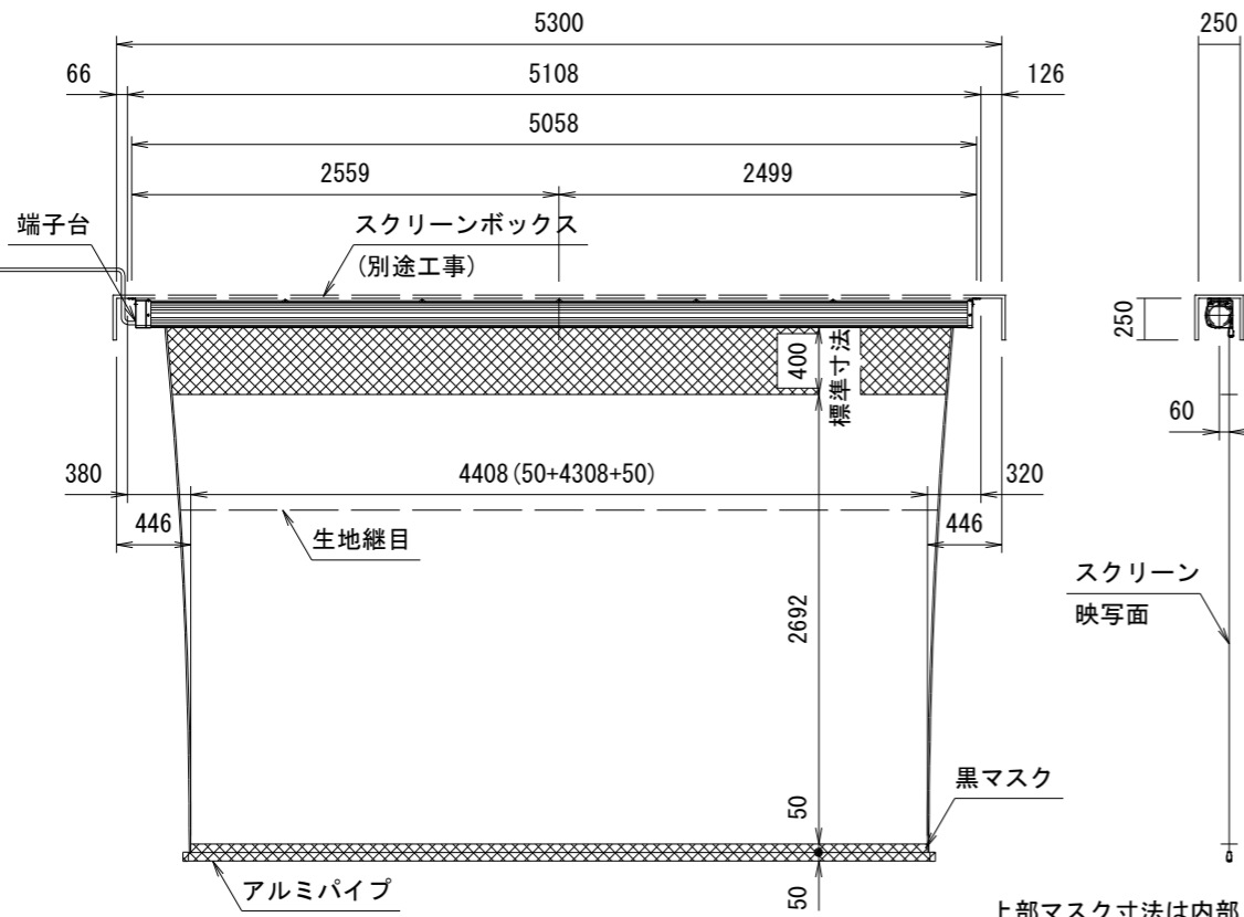
外觀図 S=1/50
