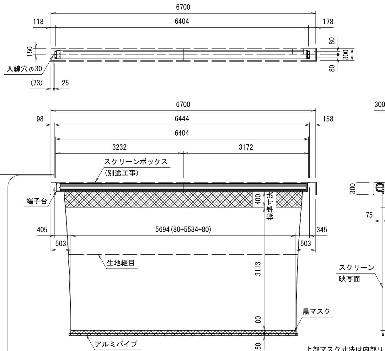
外観図 S=1/60
