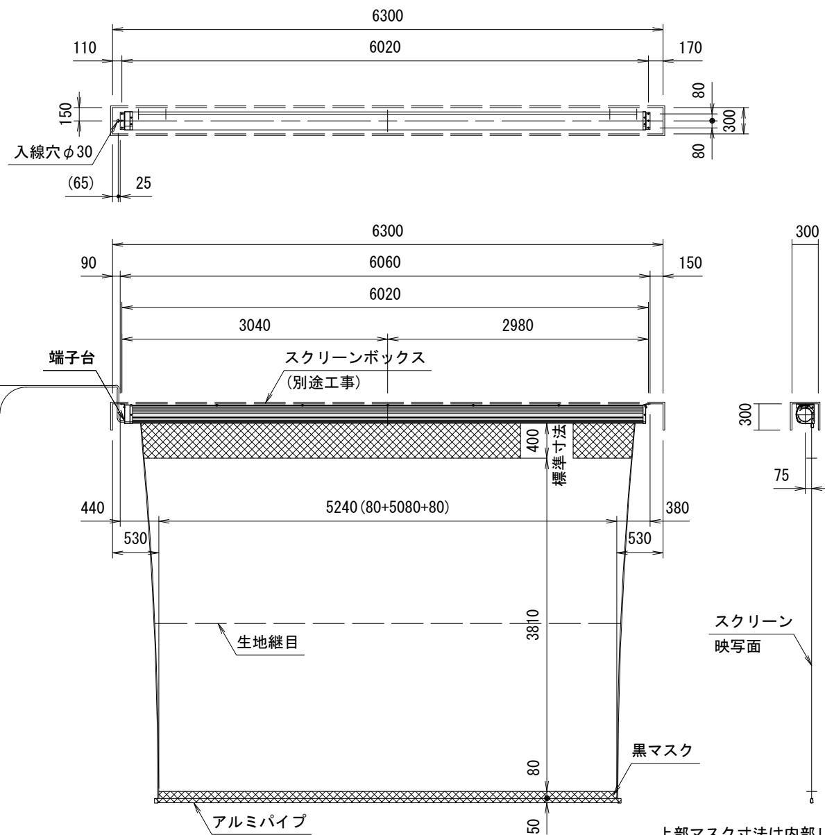
外観図 S=1/60
