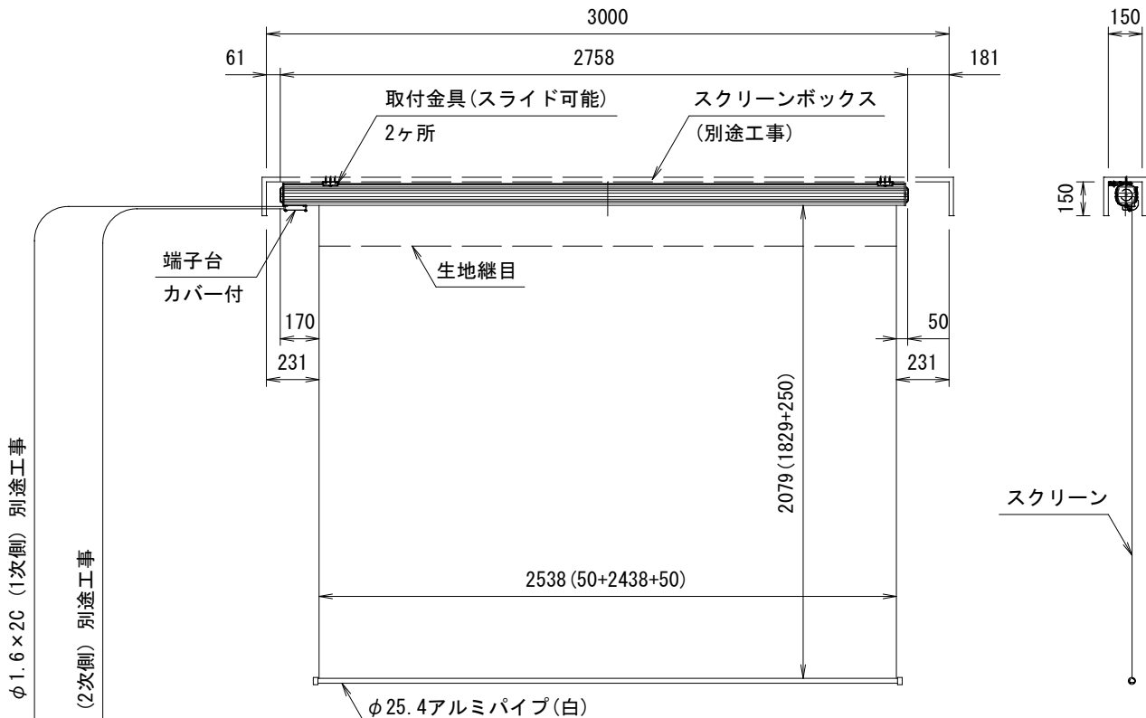
外觀図 S=1/30
