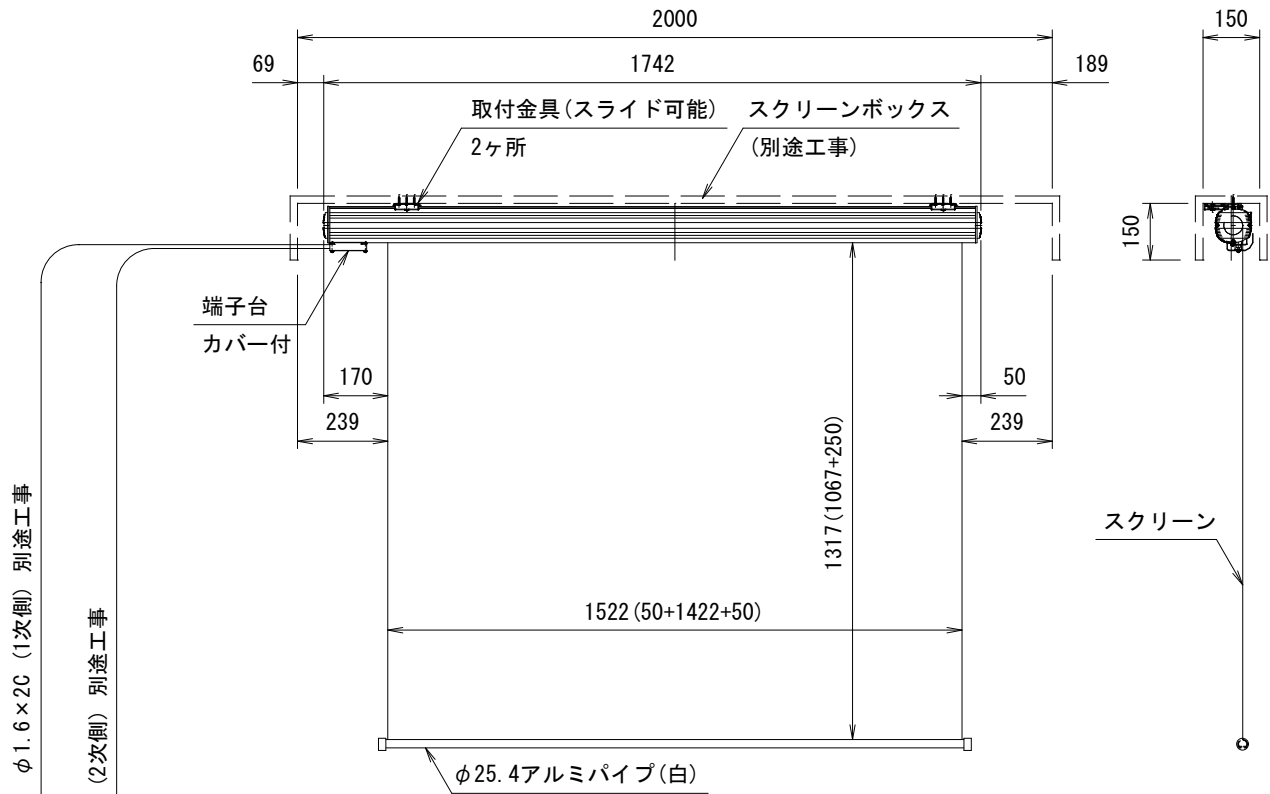
外観図 S=1/20
