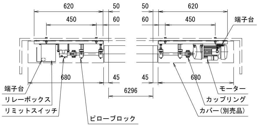
取付詳細図 S=1/20
