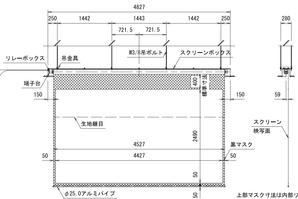
外観図 S=1/50
