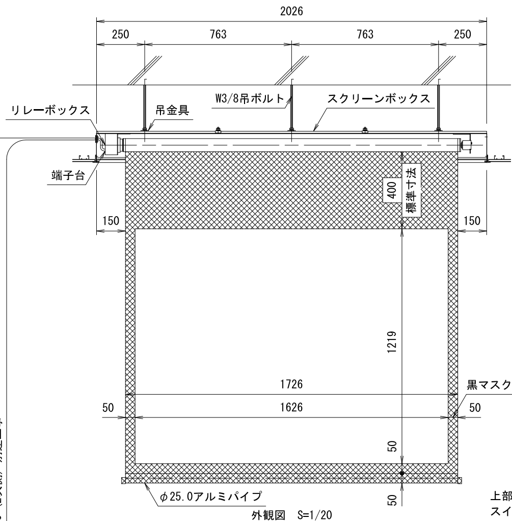
外観図 S=1/20
