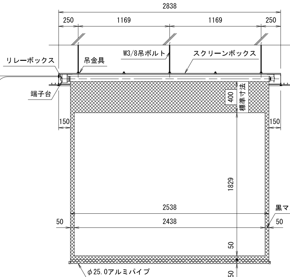
外観図 S=1/30
