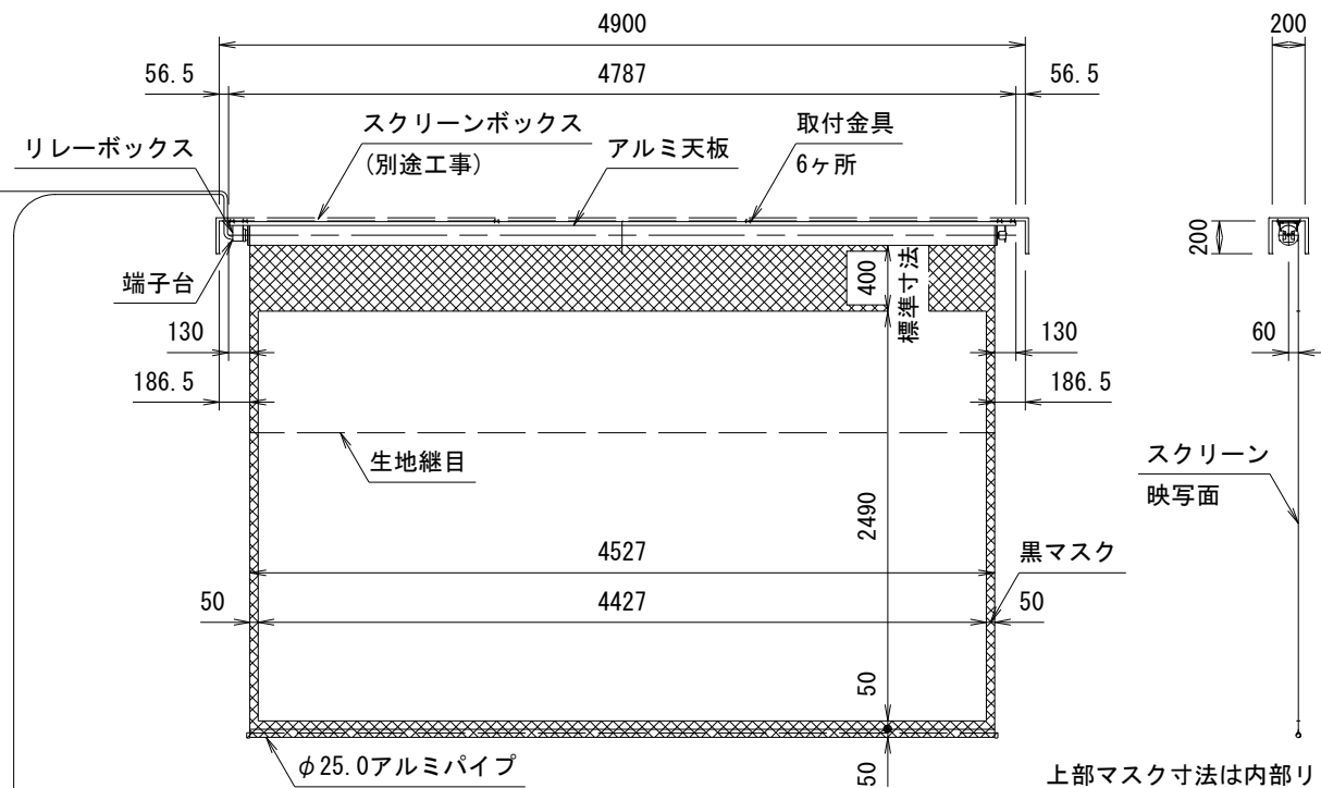
外觀図 S=1/50
