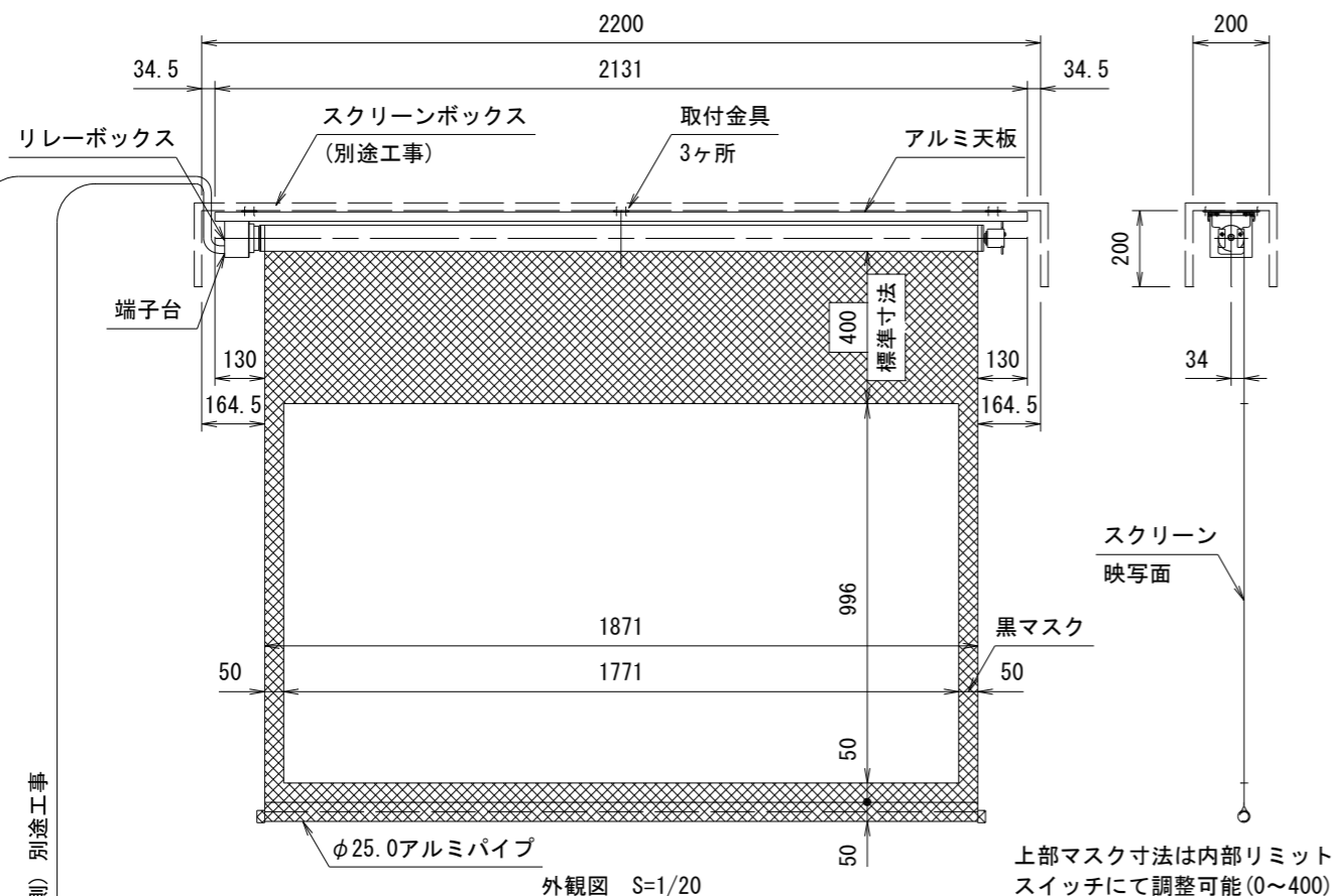
外観図 S=1/20
