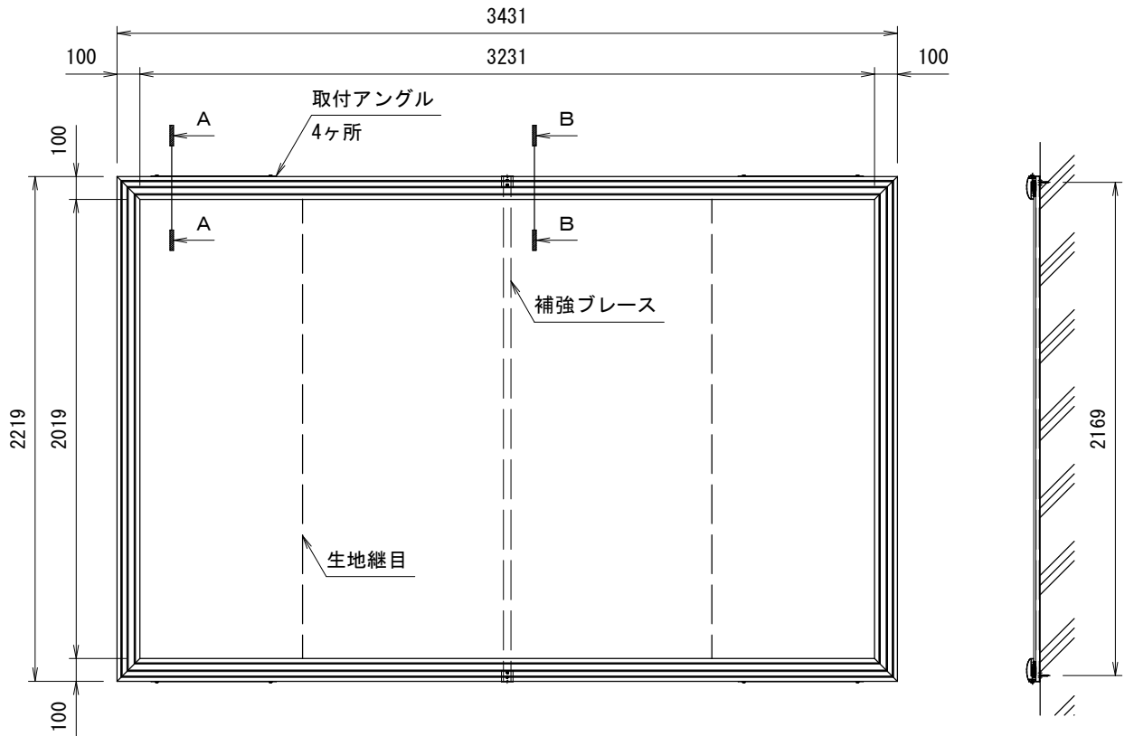
外観図 S=1/30
