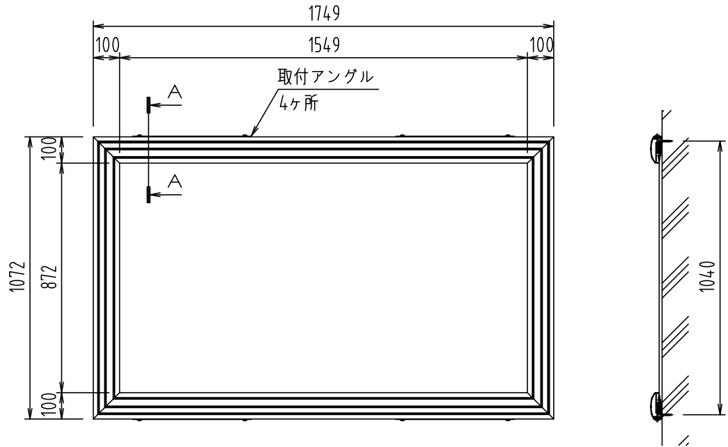
外觀図 S=1/20
