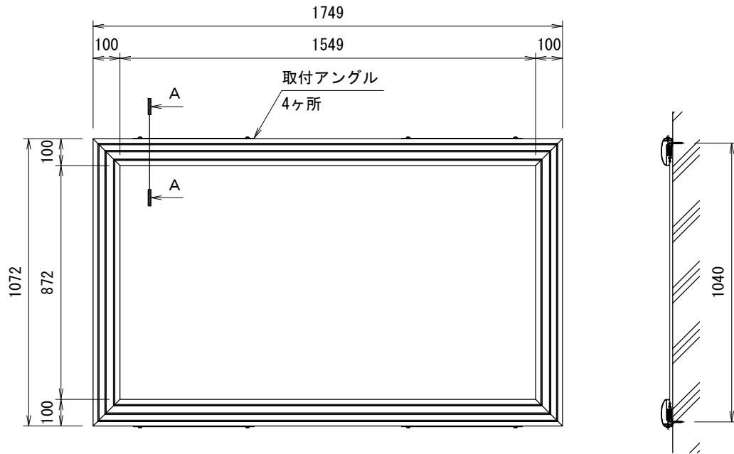
外観図 S=1/20
