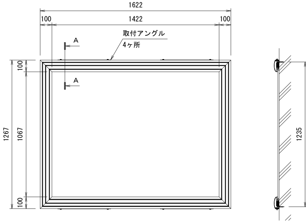
外観図 S=1/20
