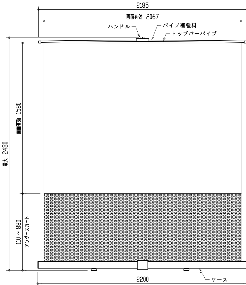
スクリーン設置図
