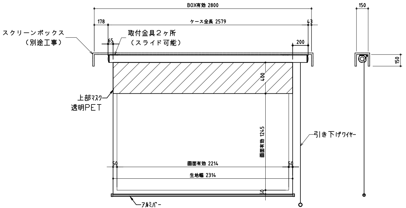
外観図 S=1/30
