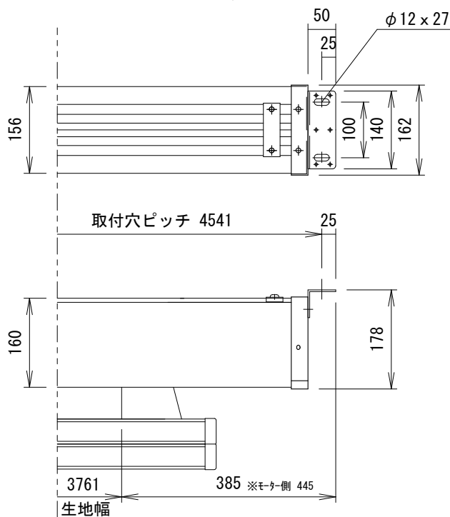
外観図 1/40
