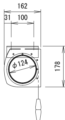
取付詳細図 1/10
