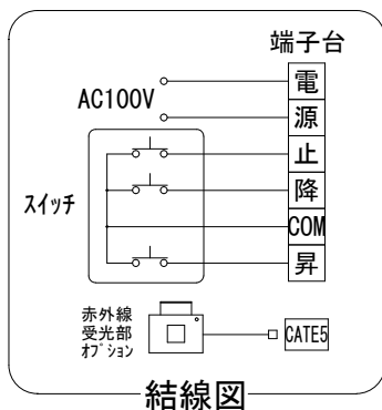
外観図 1/30
